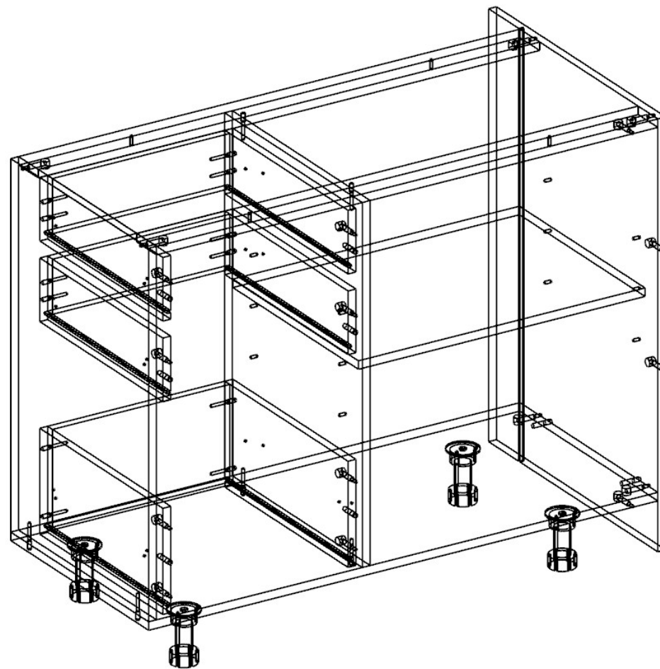
Рабочий стол с ящиками
