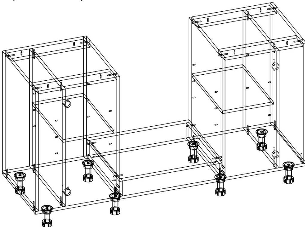
Рабочий стол с Духовым шкафом
